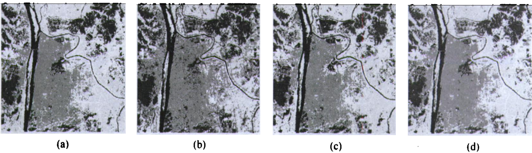
图 6 常用土地利用分类方法结果图 (a) 最大似然法; (b) 神经网络法; (c) 决策树法; (d) 纹理与光谱信息多分类器融合分类法
